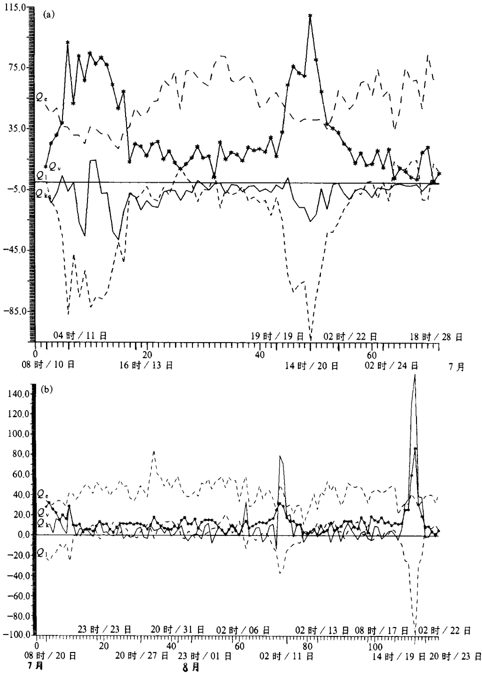
图1 海气界面热量平衡逐时变化曲线 纵坐标为海气界面热量( Q_e 、 Q_v \times 10 、 Q_l \times 10 、 Q_k , 单位: W \cdot m^{-2} ) (a) 1号浮标; (b) 4号浮标
