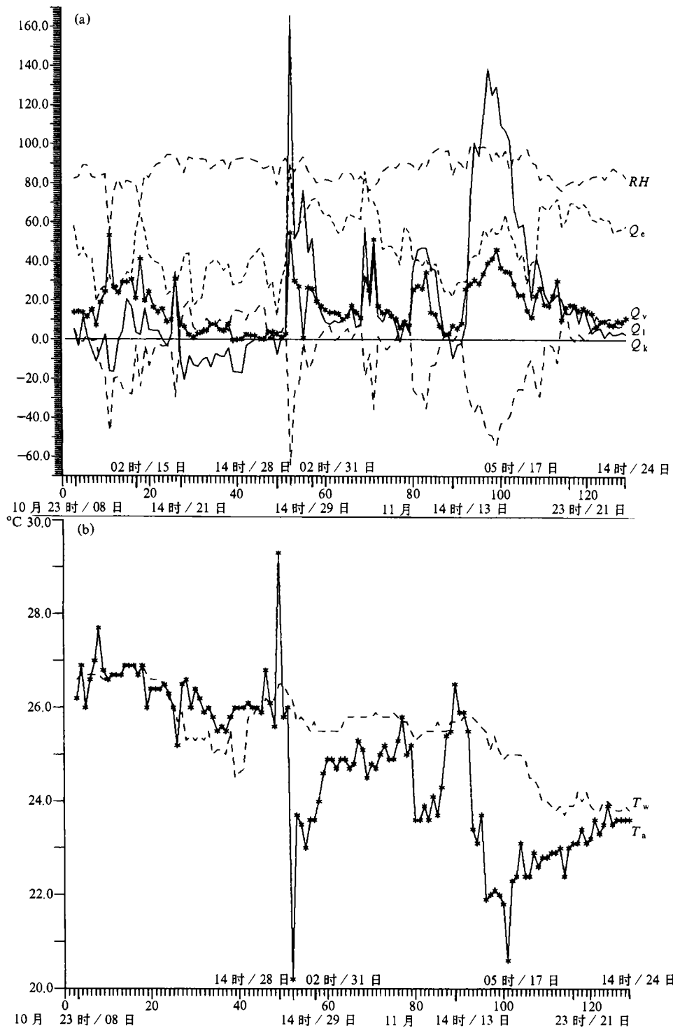
图3 海气界面热量交换、水温( T_w )和气温( T_a )逐时变化曲线
