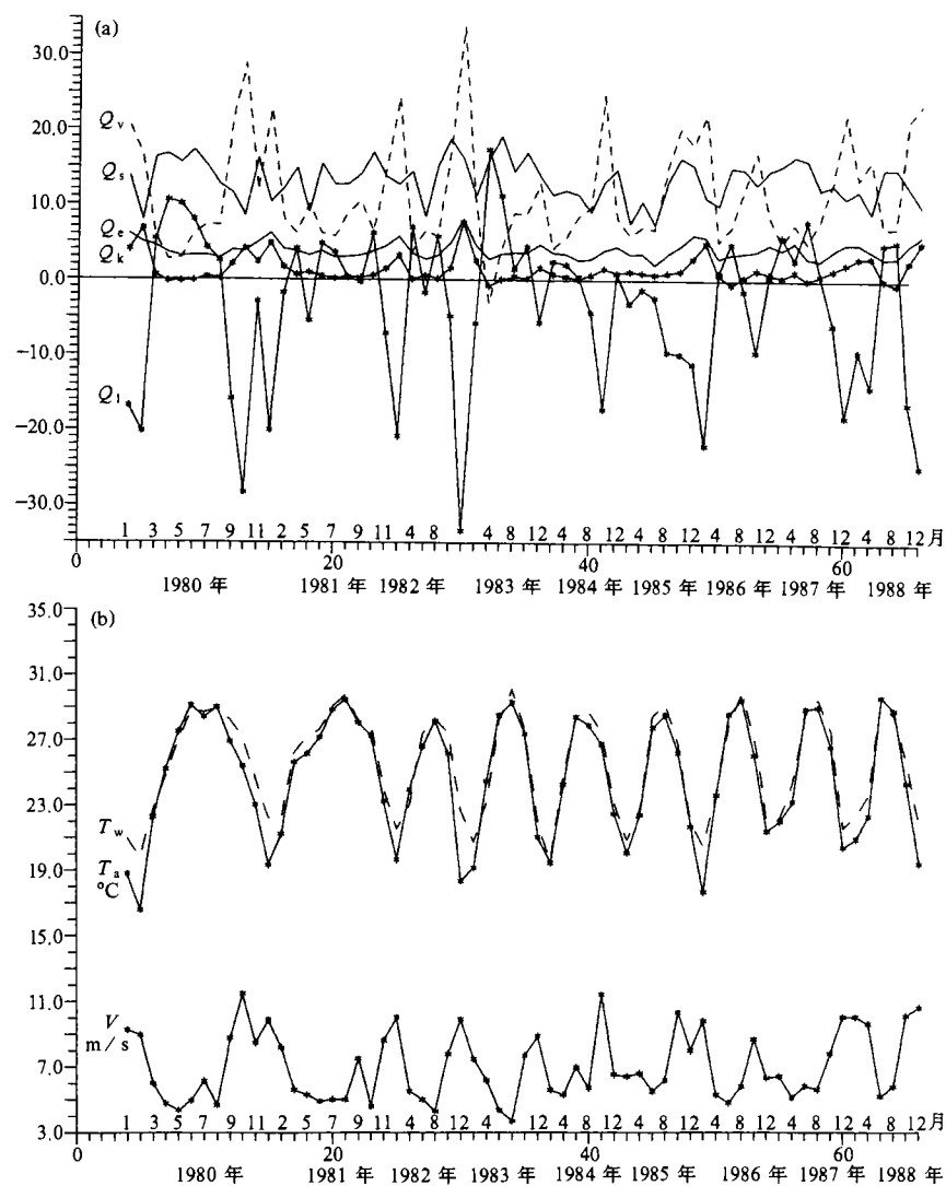
图5 南海(1980~1988年)海气界面热量交换日总量、水温、气温、风速各月日的平均值 (a) 海气界面热量交换日总量; (b) 水温( T_w ), 气温( T_a ), 风速( V ) (a) 中纵坐标为海气界面热量交换日总量( Q_s 、 Q_v 、 Q_e 、 Q_k 、 Q_i , 单位: \text{MJ} \cdot \text{m}^{-2} \cdot \text{d}^{-1} )
