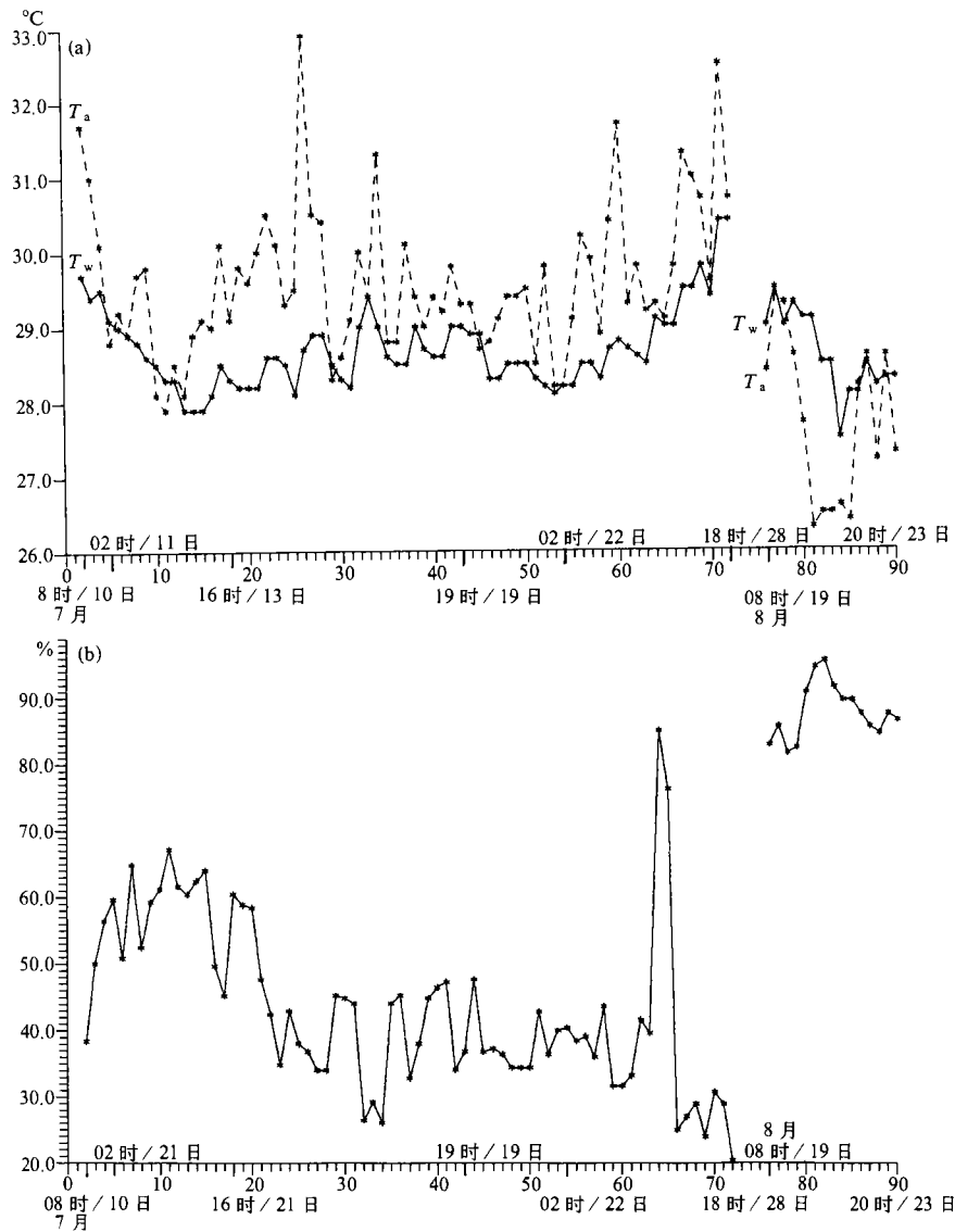
图2 水温、气温、相对湿度逐时变化曲线 (a) 水温( T_w )和气温( T_a ); (b) 相对湿度
