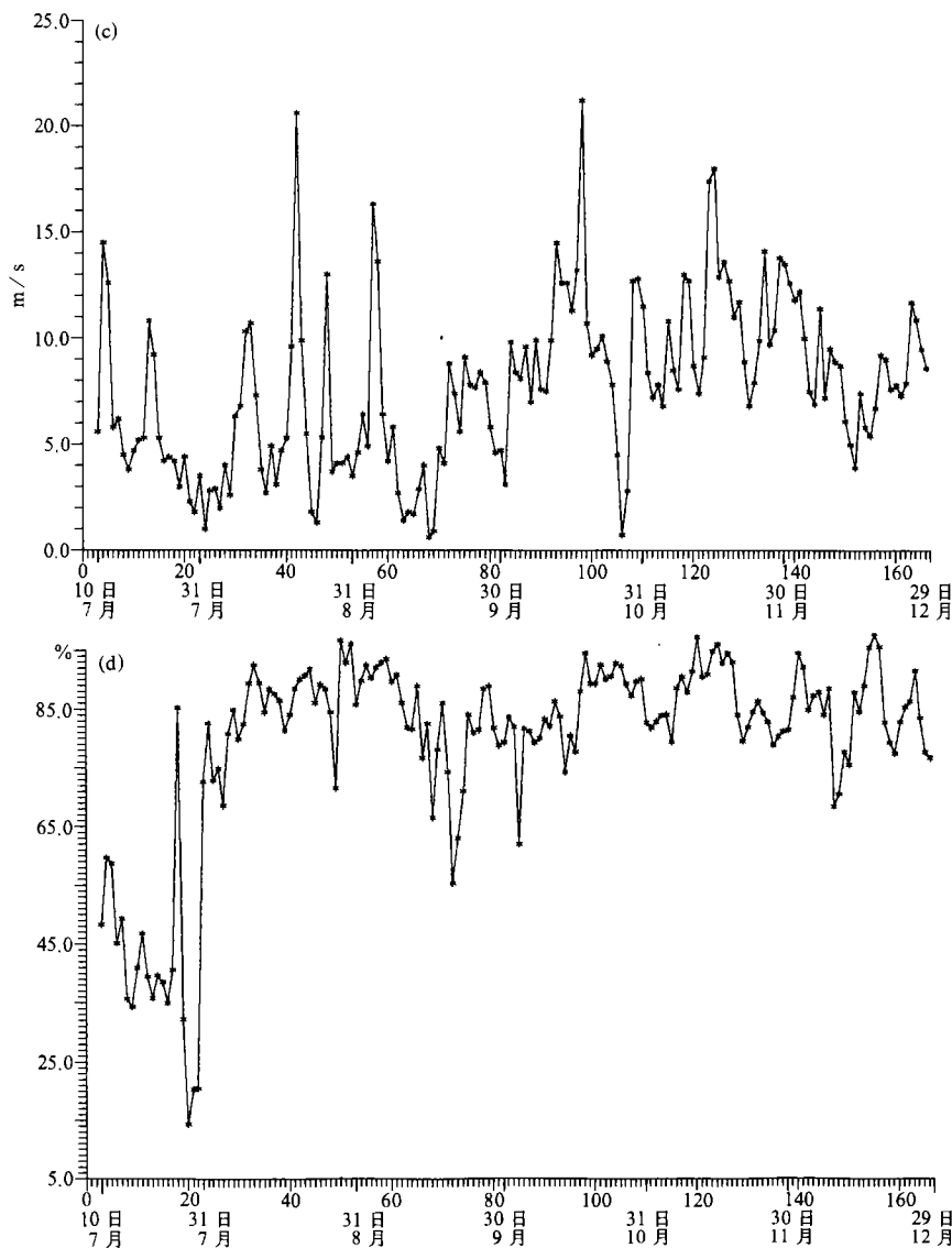
图 4 (续) 海气界面热量交换日总量、水温、气温、风速、相对湿度日平均值变化曲线 (c) 风速 ( V ); (d) 相对湿度
