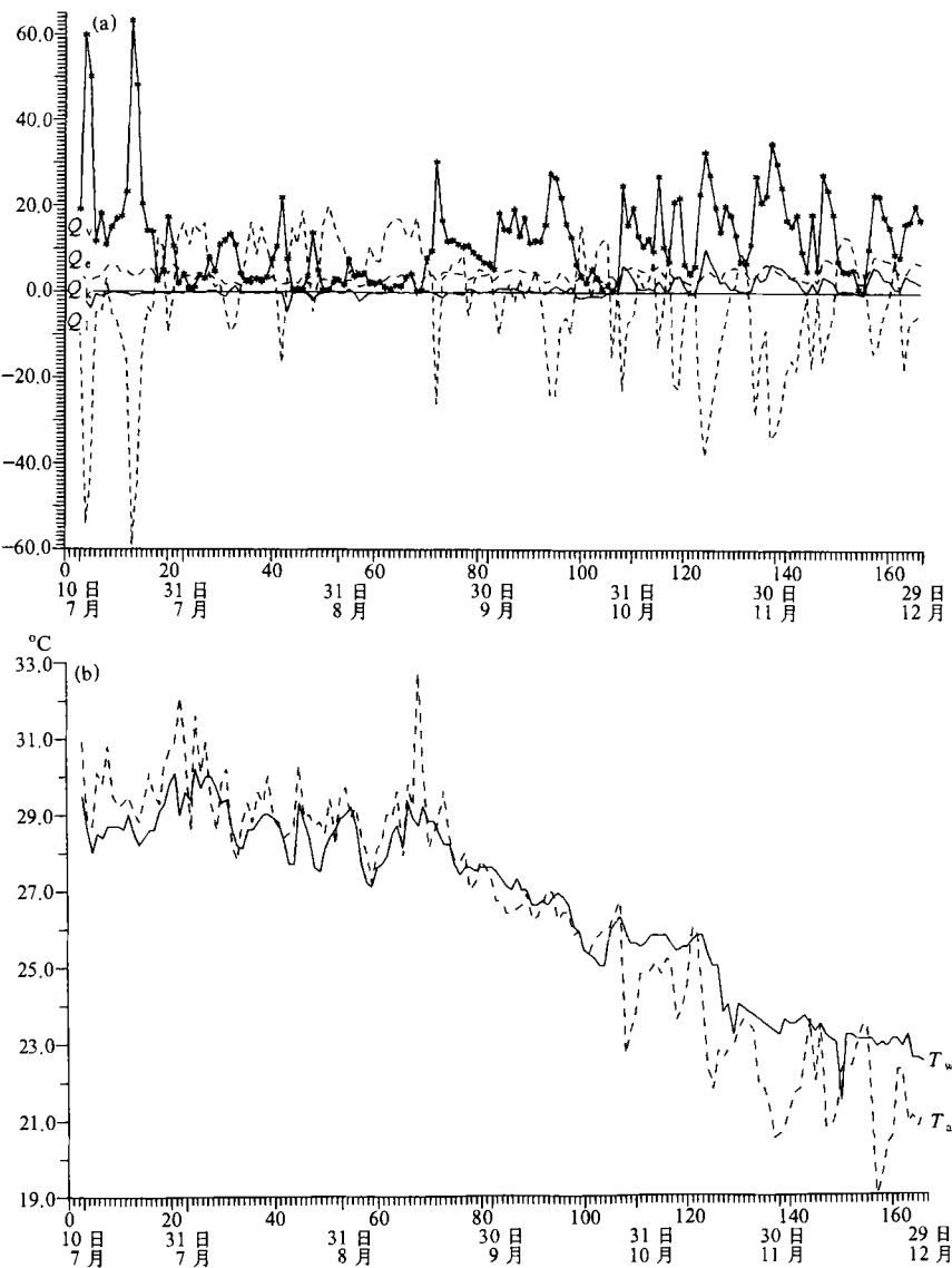
图4 海气界面热量交换日总量、水温、气温、风速、相对湿度日平均值变化曲线 (a) 海气界面热量交换日总量; (b) 水温( T_w )、气温( T_a ); (a) 中纵坐标为海气界面热量交换日总量( Q_v 、 Q_e 、 Q_k 、 Q_l , 单位: \text{MJ} \cdot \text{m}^{-2} \cdot \text{d}^{-1} )
